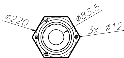
PLANTILLA DE INSTALACIÓN INSTALLATION TEMPLATE
